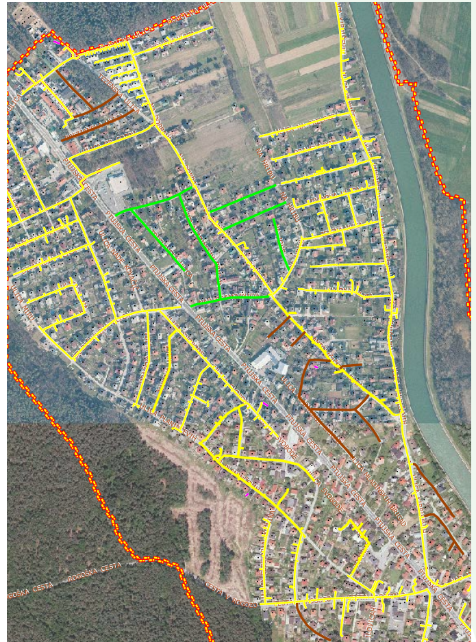
Načrt širitve plinovodnega omrežja v Miklavžu na Dravskem polju
